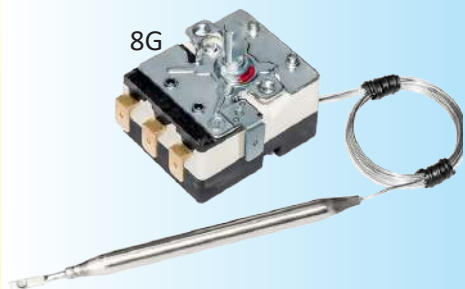
Termostato monopolar con bulbo y capilar, rangos de temperatura de hasta 500 °C
